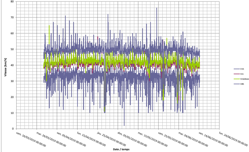
Vitesse en fonction du temps
